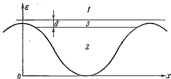
Рис. 2. Функция распределения во внешней и внутренней областях: 1 — внешняя область, 2 — внутренняя область, 3 — пограничный слой
