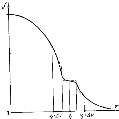
Рис. 1. Форма функции распределения при учете обратного действия волн на «фон». Вне резонансной области функция распределения — максвелловская
